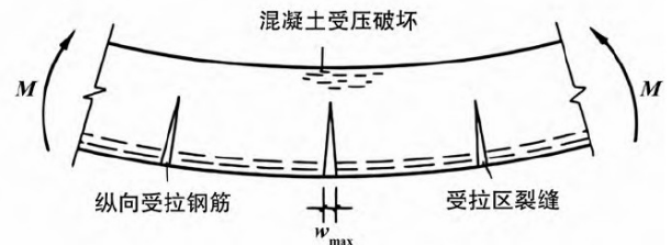
图 1 受弯裂缝形态图
