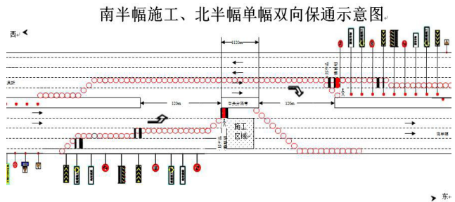
图 3 路基改桥第二阶段
