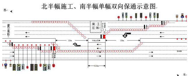
图 2 路基改桥第一阶段
