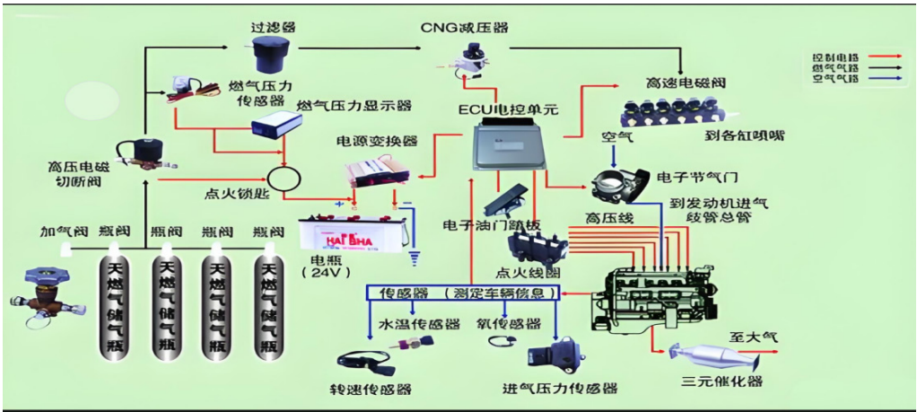
图一 汽车电子 ECU 控制单元
